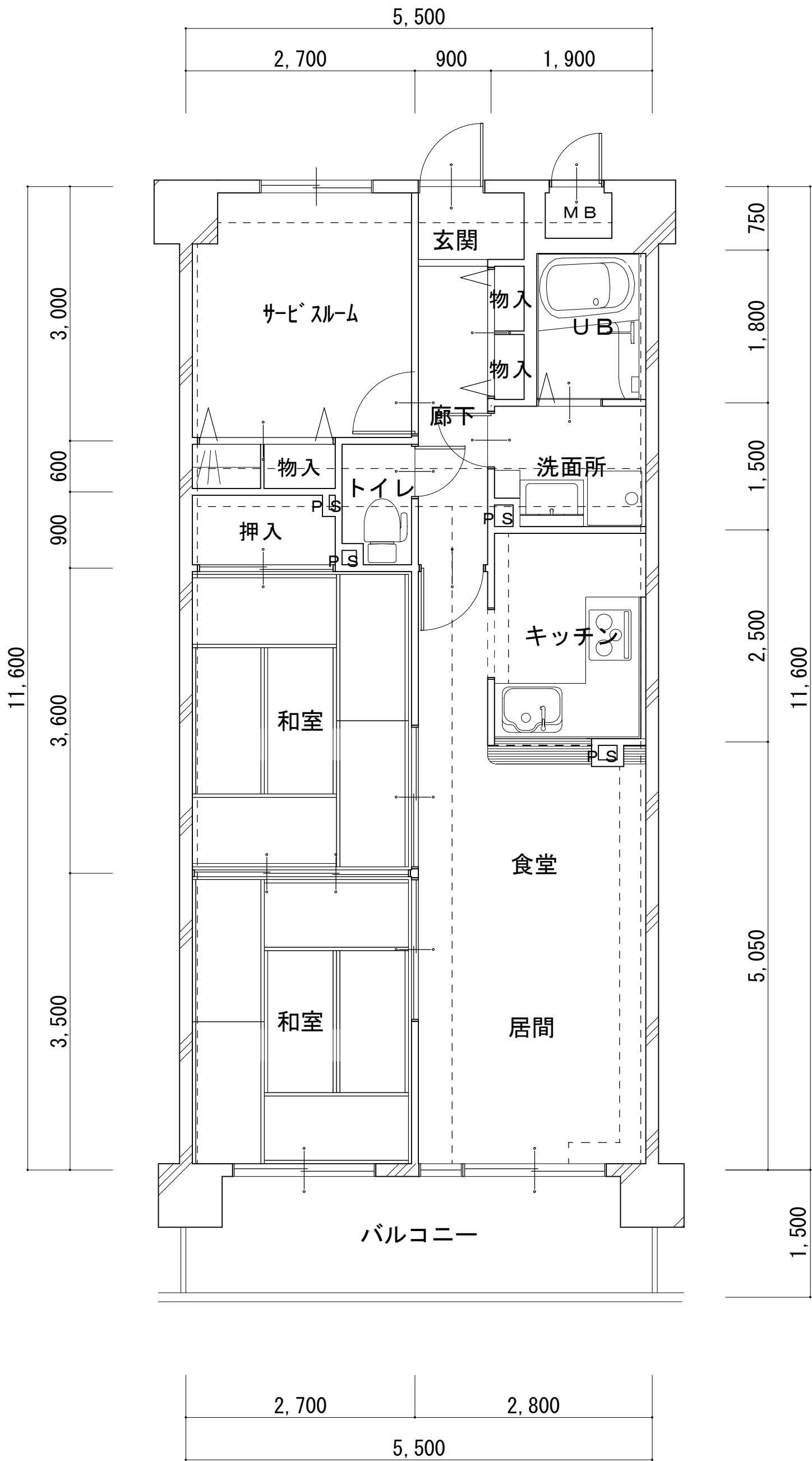
現況図
